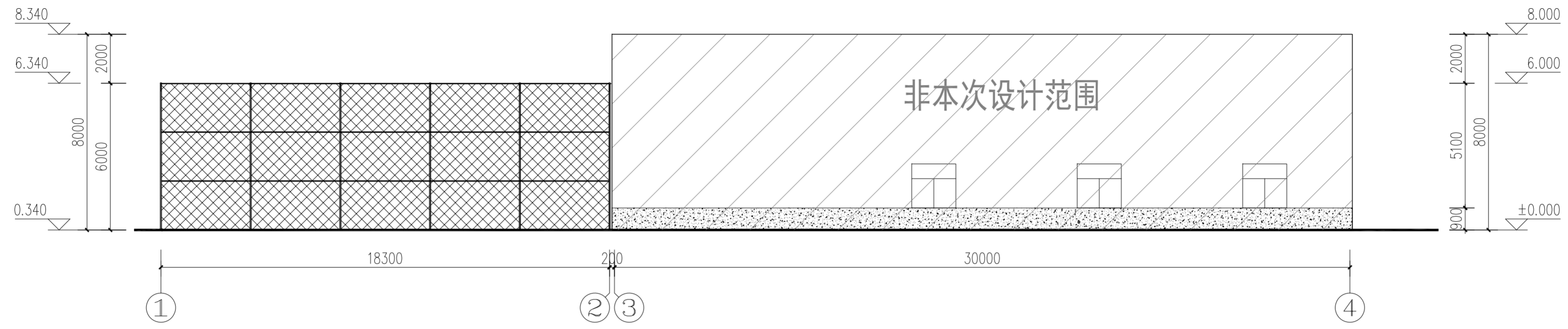
①-④轴立面图 1:100
