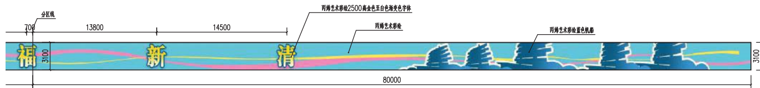
④ 飘带雕塑处BK2153+350-BK2153+750 声屏障装饰图标段五 1:200 说明：此次为右侧声屏障内侧装饰立面。
