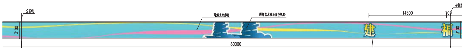
③ 飘带雕塑处BK2153+350-BK2153+750 声屏障装饰图标段四 1:200 说明：此次为右侧声屏障内侧装饰立面。
